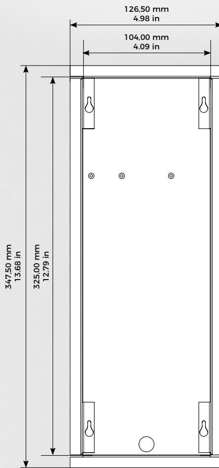
Carcasa de montaje empotrado
