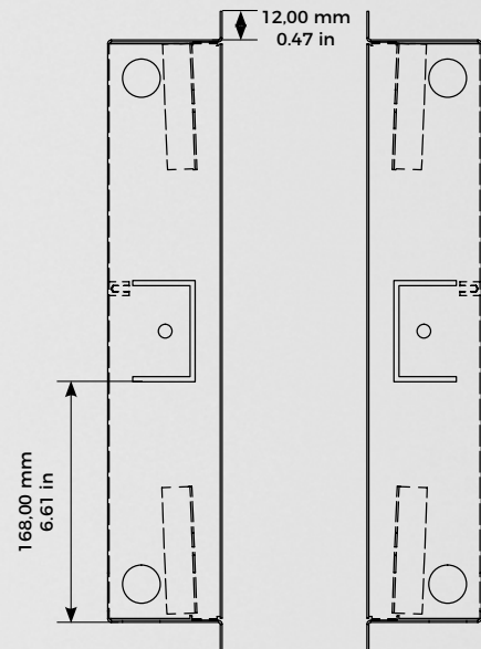
Carcasa de montaje empotrado
