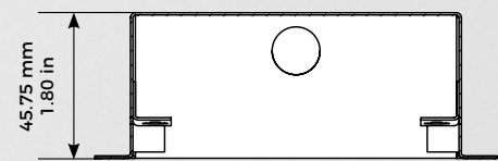
Boîtier de montage arrière (encasté)
