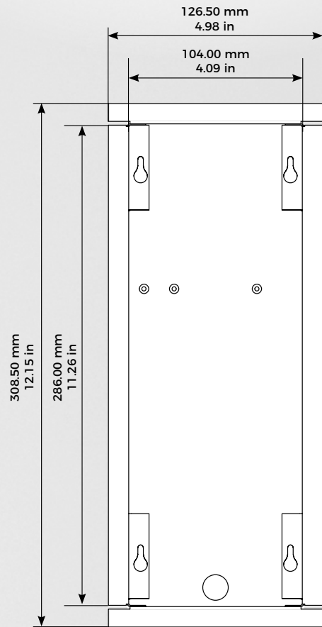
Boîtier de montage arrière (encasté)
