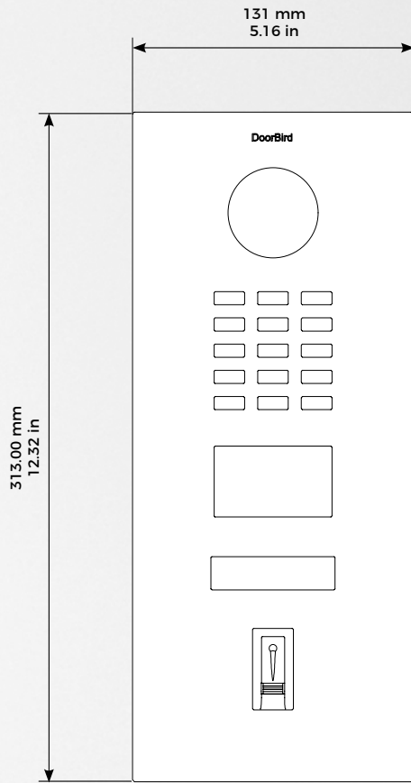
Face avant
