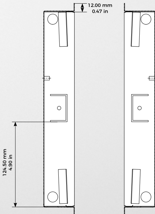
Boîtier de montage arrière (encasté)
