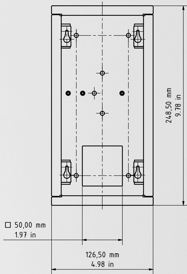
Carcasa de montaje empotrado
