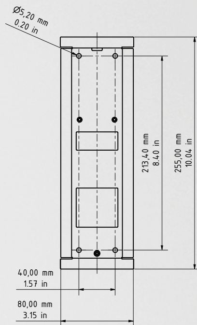
Unterputzgehäuse
