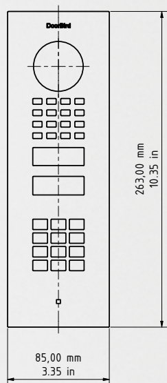
Frontblende
