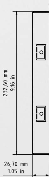
Frontblende
