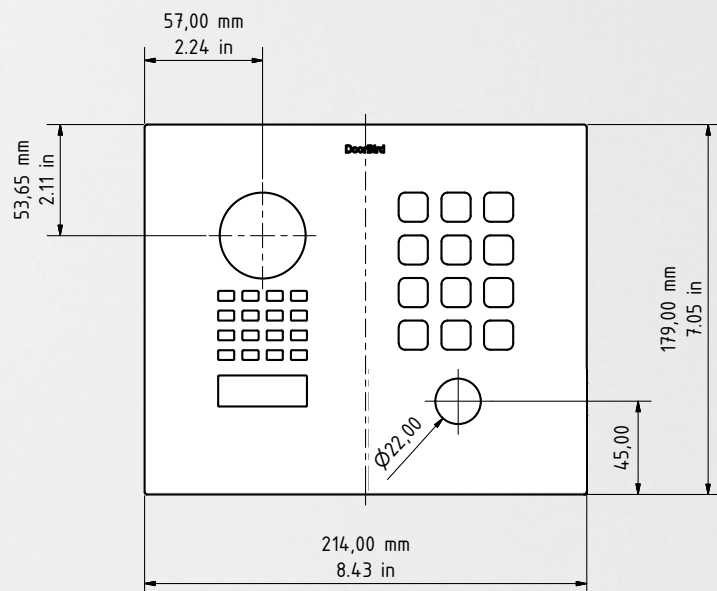
Face avant
