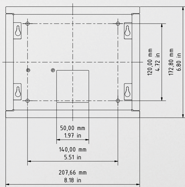
Boîtier de montage arrière (encasté)
